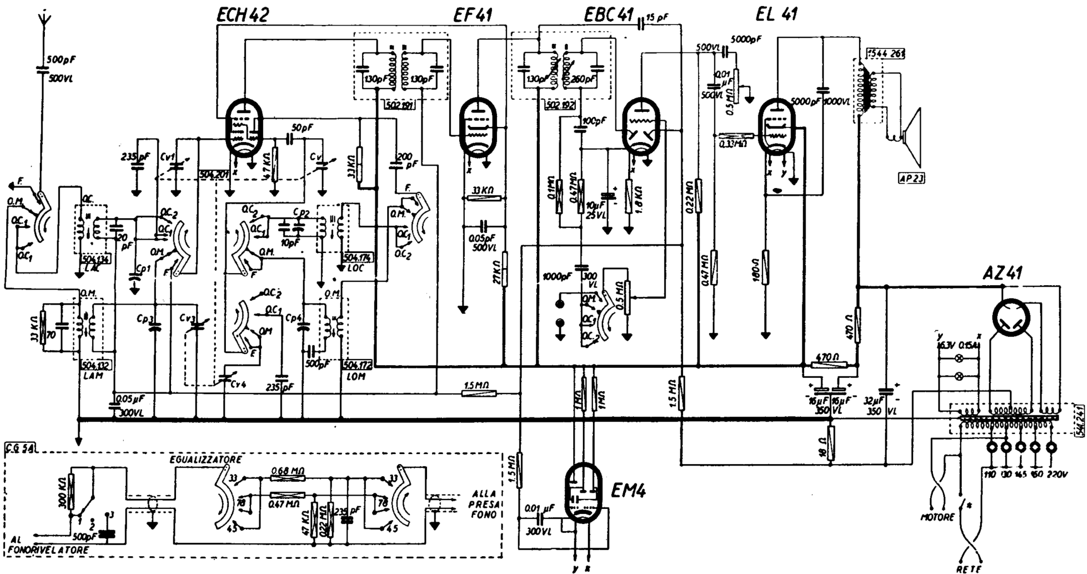
VOCE DEL PADRONE - FONORADIO mod. 1545. Onde medie e 2 gamme espanse onde corte. Media frequenza 465 kc/s. Potenza indistorta di uscita 3 watt. Consumo 45 watt.
